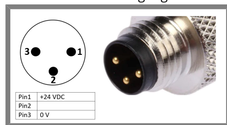
Steckerbelegung
