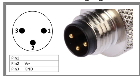
Steckerbelegung
